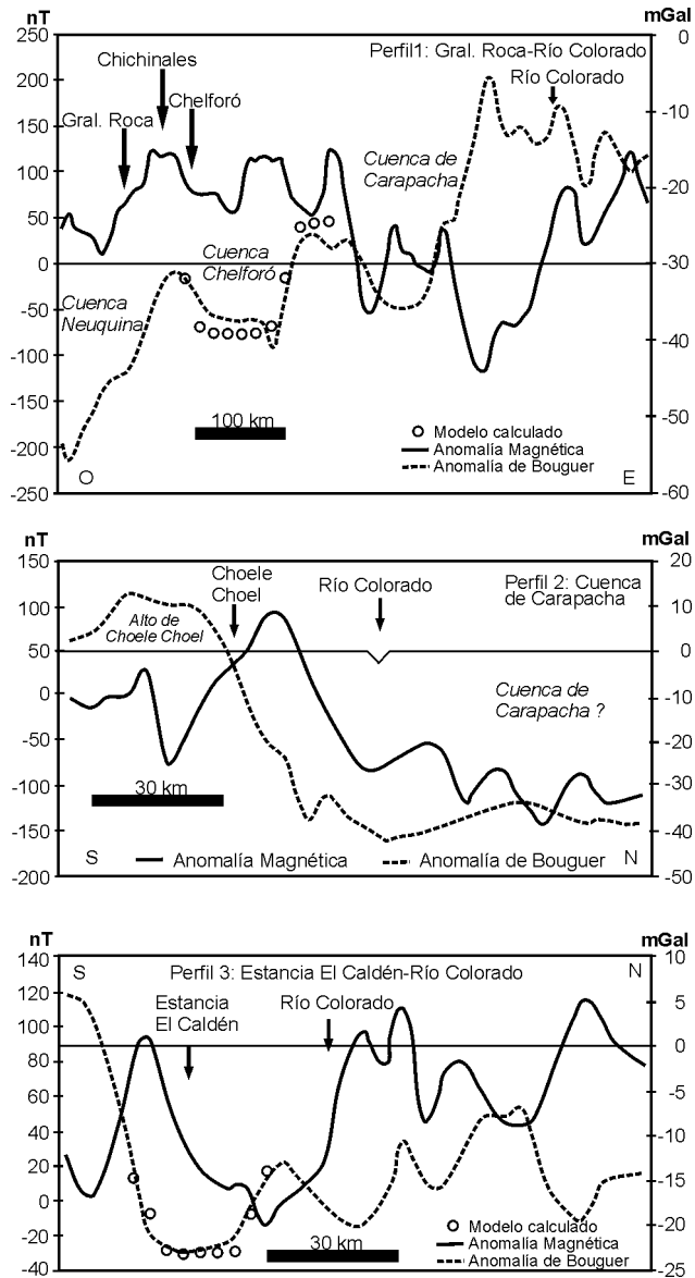
Figura 5: Perfiles gravimagnetométricos. Perfil 1. General Roca – Río Colorado; Perfil 2. Cuenca de Carapacha; Perfil 3. Estancia El Caldén – Río Colorado
