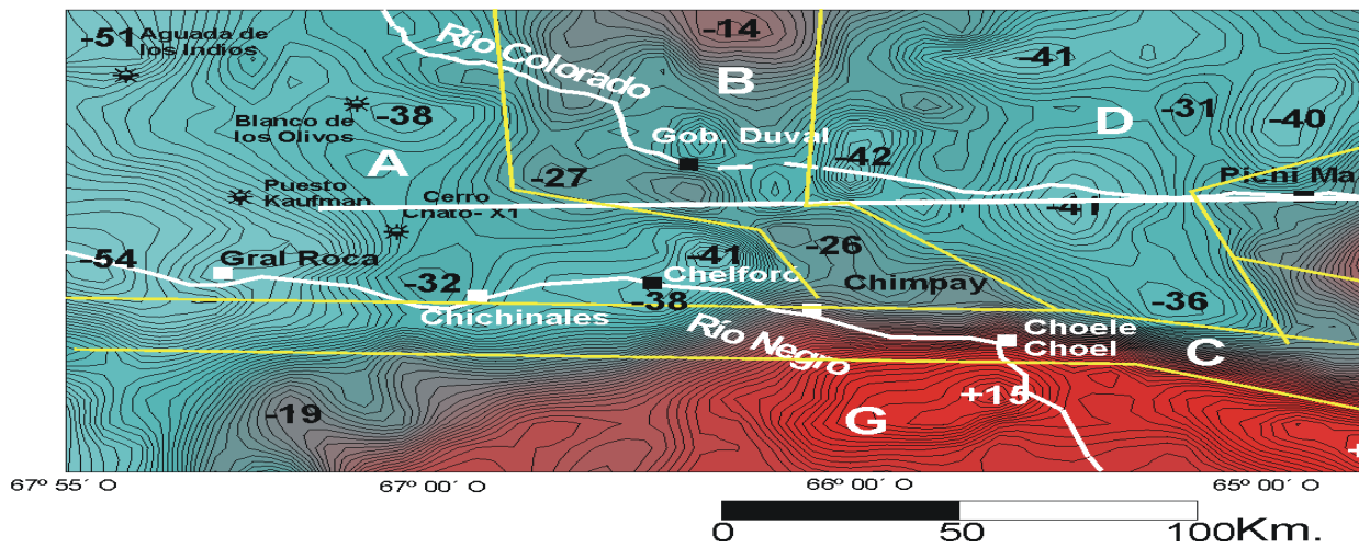
Figura 4: Mapa de anomalías gravimétricas de Bouguer y zonas seleccionadas por sus singularidades geológicas y geofísicas.
