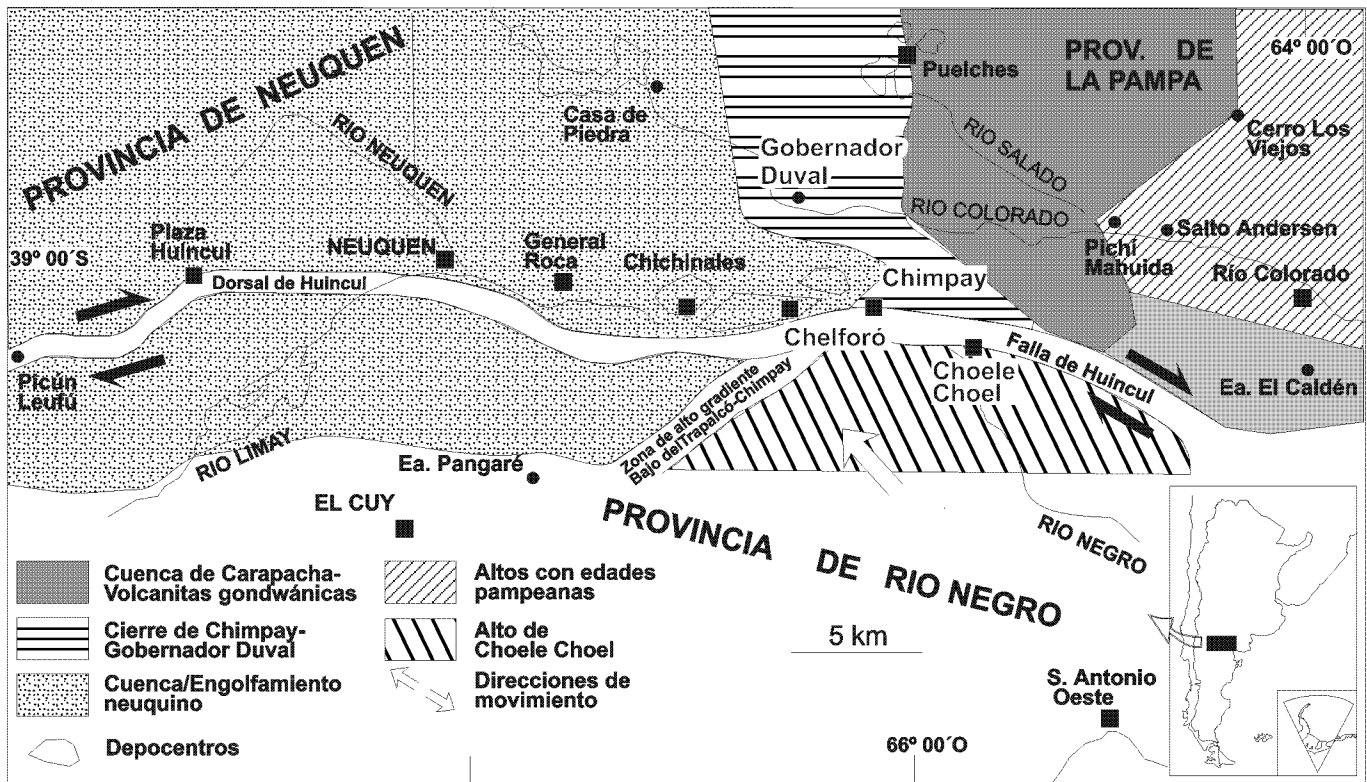
Figura 6: Configuración geológica basado en las interpretaciones geofísicas en el sector norte de la provincia de Río Negro.
