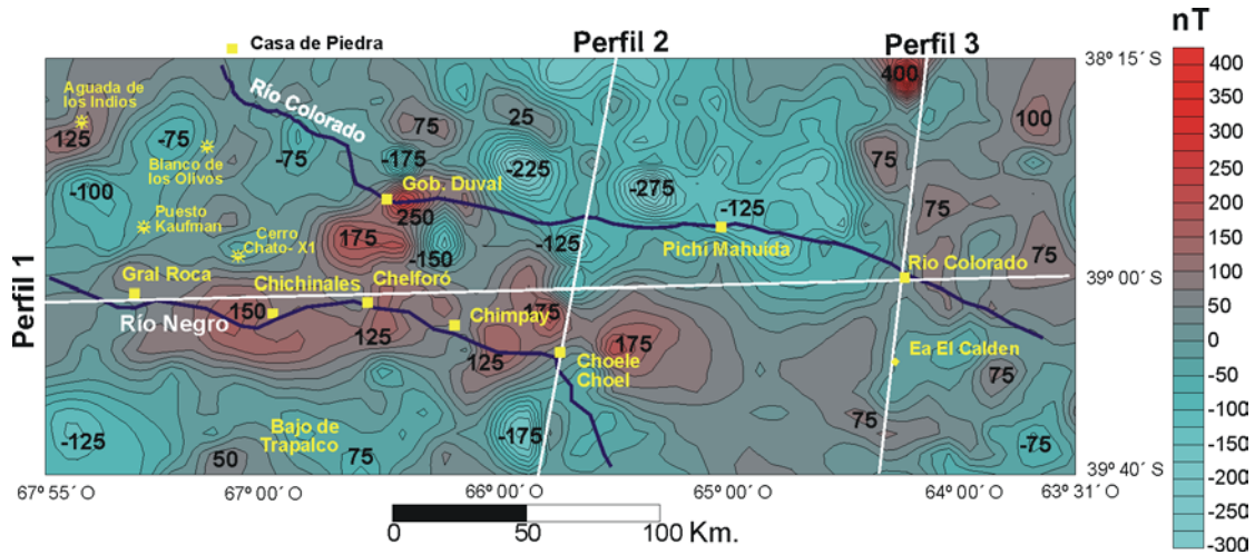
Figura 3: Mapa de anomalías del campo magnético terrestre, isolíneas cada 25 nT.
