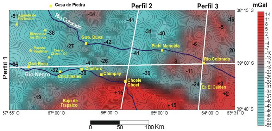
Figura 2: Mapa de anomalías gravimétricas de Bouguer y ubicación de perfiles. Isolíneas cada 1 mGal.
