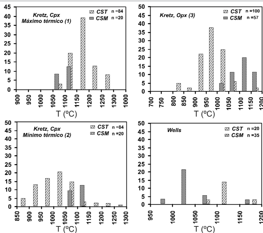
Figura 4: Histogramas de frecuencia de temperaturas calculadas mediante la termometría ortopiroxeno-clinopiroxeno usando los termómetros de Kretz (1982) para piroxenos cálcicos, mostrando consecuentemente las máximas (arriba a la izquierda) y mínimas (abajo a la izquierda) temperaturas obtenidas, termómetros de Kretz (1982, derecha arriba) y de Wells (1977, derecha abajo) para el intercambio de Fe-Mg en piroxenos pobres en calcio.
