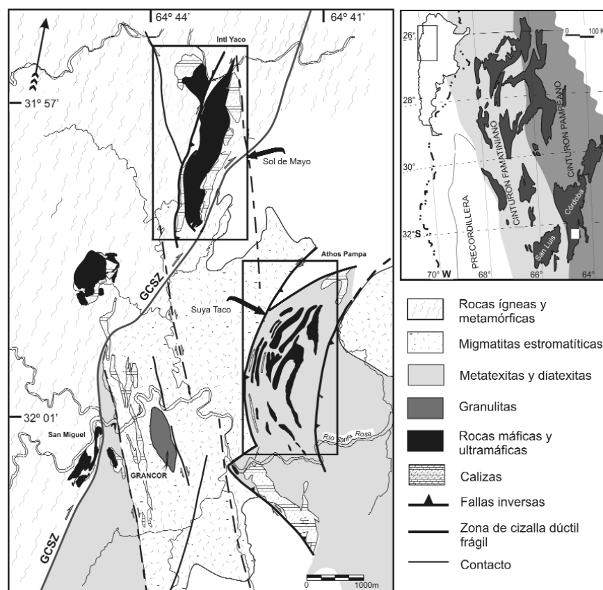
Figura 1: Mapa geológico mostrando la ubicación de los Complejos Sol de Mayo y Suya Taco en el norte de las Sierras de Comechingones. A la derecha se incluye el contexto geológico de las Sierras Pampeanas; la distribución de los cinturones orogénicos corresponde a Rapela et al. (1998).
