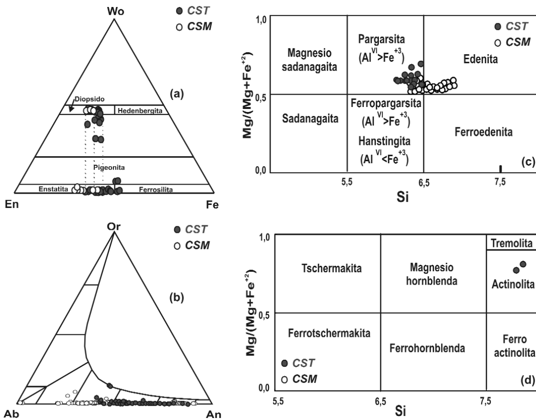
Figura 3: a) Proyección de piroxenos en el diagrama Wo-En-Fs de clasificación propuesto por Morimoto et al. (1989) para la clasificación de piroxenos ferromagnesianos y cálcicos, las líneas representan estabilidad entre pares clinopiroxenos y ortopiroxenos. b) Diagrama Ab-An-Or donde se muestra la variación composicional observada las plagioclasas presentes en las rocas máficas de ambos complejos. (c-d) Diagramas de clasificación de anfíboles según Leake et al. (1997). c) Corresponde a anfíboles con Ca > 1,5 c.p.f.u. y (Na+K)A > 0,5 c.p.f.u. d) Corresponde a anfíboles con Ca > 1,5 c.p.f.u. y (Na+K)A < 0,5 c.p.f.u.
