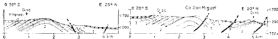
Fig. 1a. — La estructura de los cerros San Miguel (Cerrillos). 1. Precámbrico; 2. formación Mojotoro; 3. Horizonte Calcáreo-dolomítico
