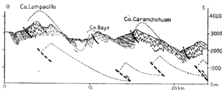
Fig. 11. — Supuesta relación entre la estructura de plegamiento de la cubierta sedimentaria y la estructura en bloque del basamento, que se ha imaginado en el perfil inferior.
