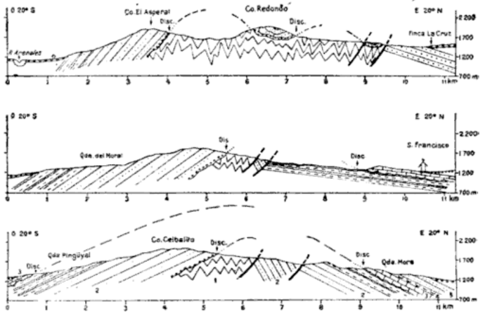
Fig. 14. — Serie de perfiles al sur de la sierra de Mojotoro. 1. Precámbrico; 2. formación Mojotoro; 3. Horizonte Calcareo-dolomítico; 4. formación Santa Bárbara; 5. formación Caralhuasi.
