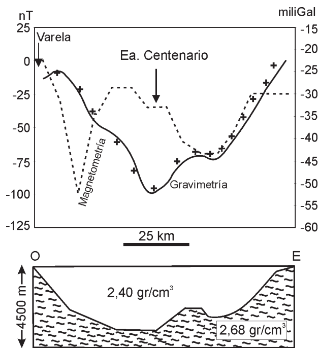
Figura 5: Perfil gravi-magnetométrico Paraje Varela – límite San Luis/Córdoba a la altura de Villa Valeria. Parte superior: curvas observadas y los valores obtenidos con el modelado geofísico presentado en la parte inferior.
