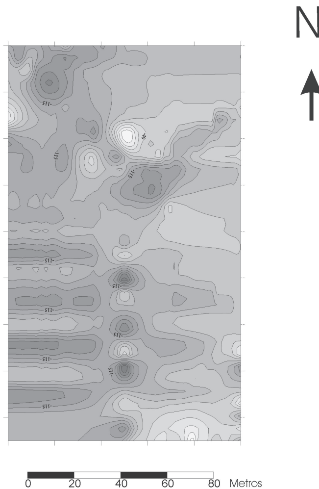
Figura 2: Mapa de anomalías magnéticas. Las curvas de isonivel se indican en gammas (= nanotesla)
