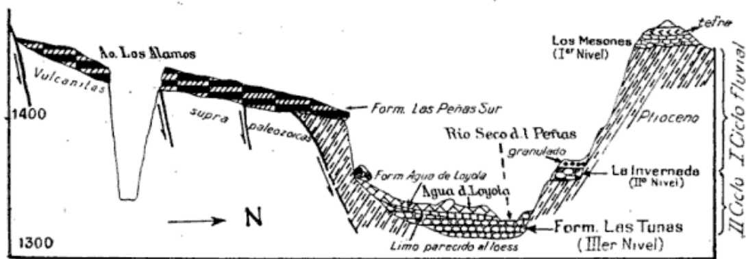
Perfil N° 6. — Las Peñas Sur
