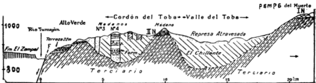
Perfil N° 18. Valle del Toba (parte boreal)
