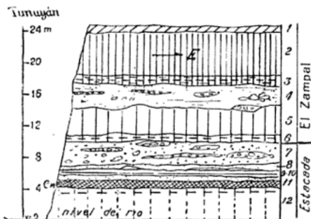
Perfil N° 20. La Estacada
