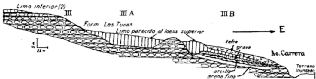
Perfil No 26. Estancia La Carrera Vieja
