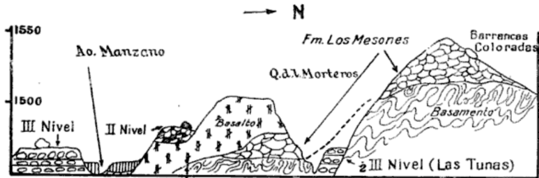
Perfil No 5. — Relaciones del basalto del Pleistoceno inferior con los niveles de pie de sierra en el Campo de Remonta «General Las Heras»
