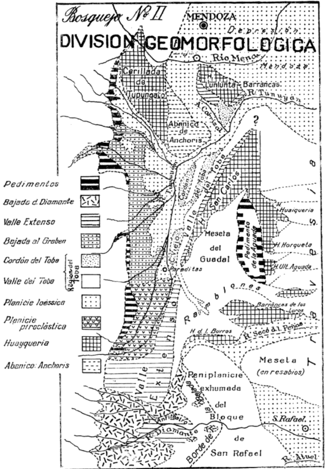
Bosquejo N° II
