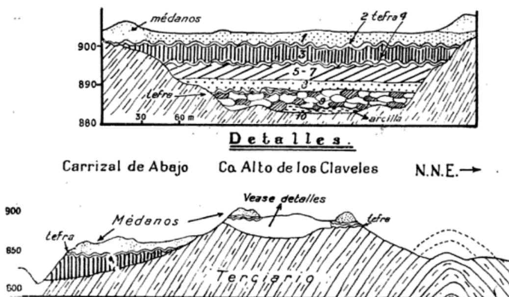
Perfil No 19. Co. Alto de los Claveles
