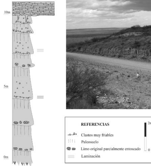
Figura 6. a) Perfil esquemático de la Formación Cerro Azul en el cerro Patagua (ubicación en Fig. 1); b) vista de los afloramientos.
