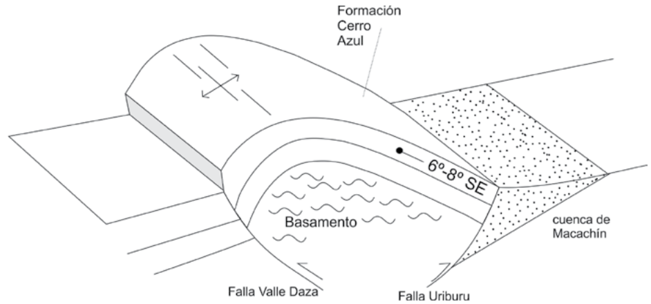
Figura 15. Pliegue propuesto para el Bloque de La Pampa Central con la ubicación de los diques clásticos en el eje de la charnela.
