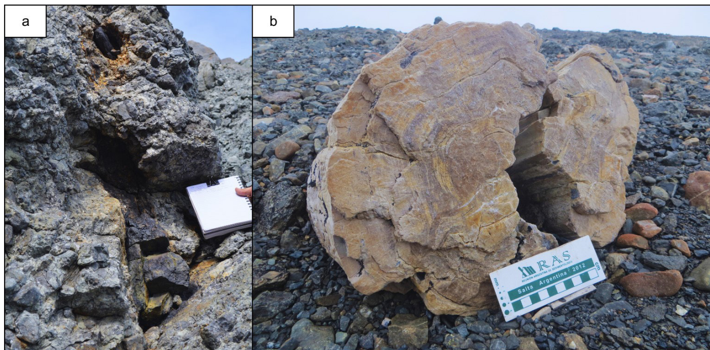
Figura 13. (a) Brecha volcánica del Grupo Volcánico Antarctic Peninsula conteniendo grandes restos de troncos; (b) Tronco en conglomerados del Miembro La Pera mostrando anillos de crecimiento bien definidos.
