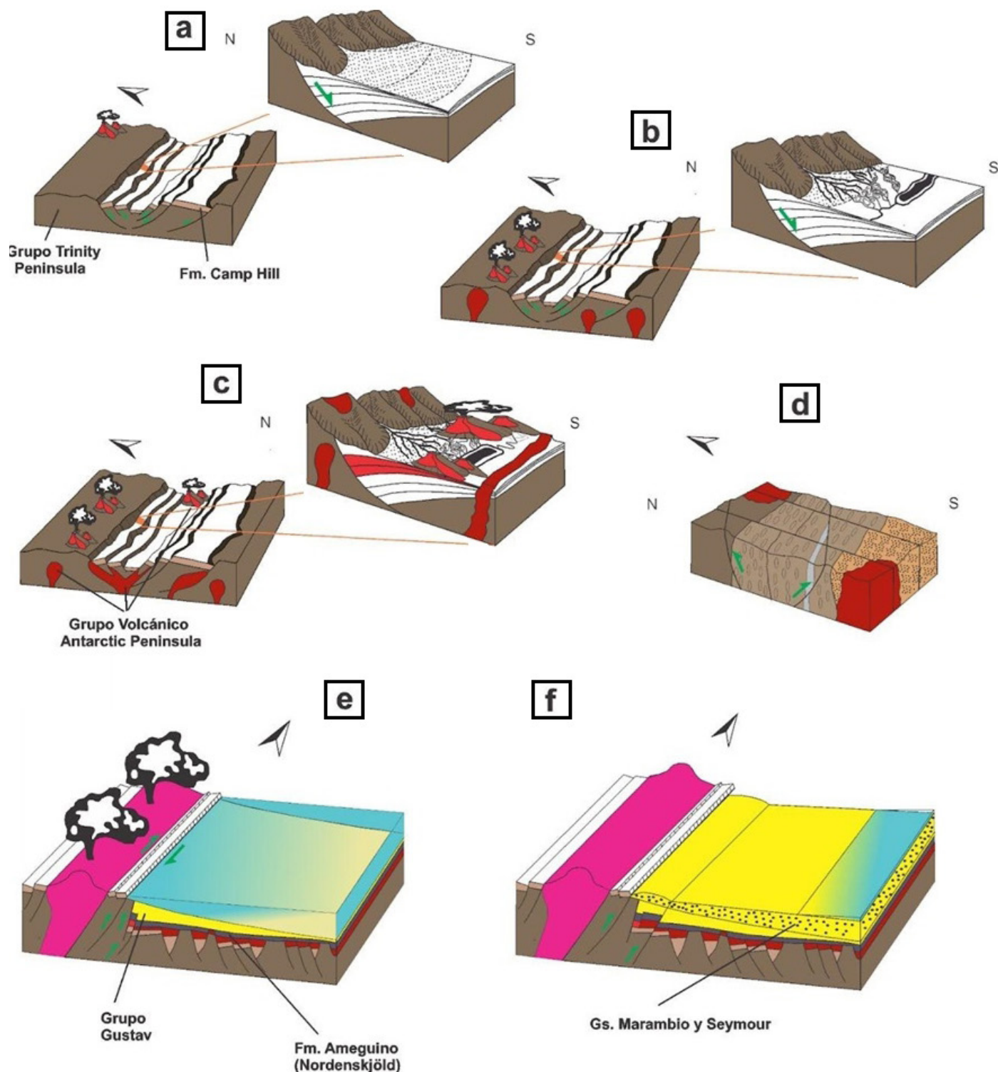
Figura 17. Modelo simplificado de la evolución del sector norte de la península Antártica. El recuadro color naranja indica la posición de la península Camp Hill. (a) Desarrollo de un sistema de rift asociado a la ruptura de Gondwana, y deposición del Miembro Dúo de la Formación Camp Hill en forma de abanicos aluviales dentro de hemigrábenes (Jurásico Medio); (b) Evolución del sistema sedimentario con desarrollo de sistemas fluviales axiales y lagos de los miembros Orca y La Pera inferior dentro de los hemigrábenes (Jurásico Medio); (c) Reactivación de las fallas de rift con la sedimentación de los miembros La Pera superior y Cascada, y migración del vulcanismo hacia el interior de los hemigrábenes con la acumulación del Grupo Volcánico Antarctic Peninsula (Jurásico Medio Tardío); (d) Reactivación compresiva de las estructuras E-O por compresión en sentido norte-sur. Se invierten las fallas del rift (Berriasiano–Barremiano); (e) Deformación de rumbo NE-SO en el Cretácico Temprano por movimiento a lo largo de un límite de placa o falla transcurrente ubicado en el borde oriental de la península Antártica. Formación de la cuenca James Ross en el Cretácico Temprano alto. Grandes fallas inversas NE a lo largo del canal Príncipe Gustavo y erosión de las sedimentitas jurásicas en el margen de la cuenca, un arco volcánico orientado NE-SO (Aptiano); (f) Inversión parcial de la cuenca de James Ross (Coniaciano en adelante) y migración de la cuña clásica hacia el este. Nótese el cambio en la orientación respecto del N geográfico en los paneles “e” y “f”, que fueron modificados de Hathway (2000).
