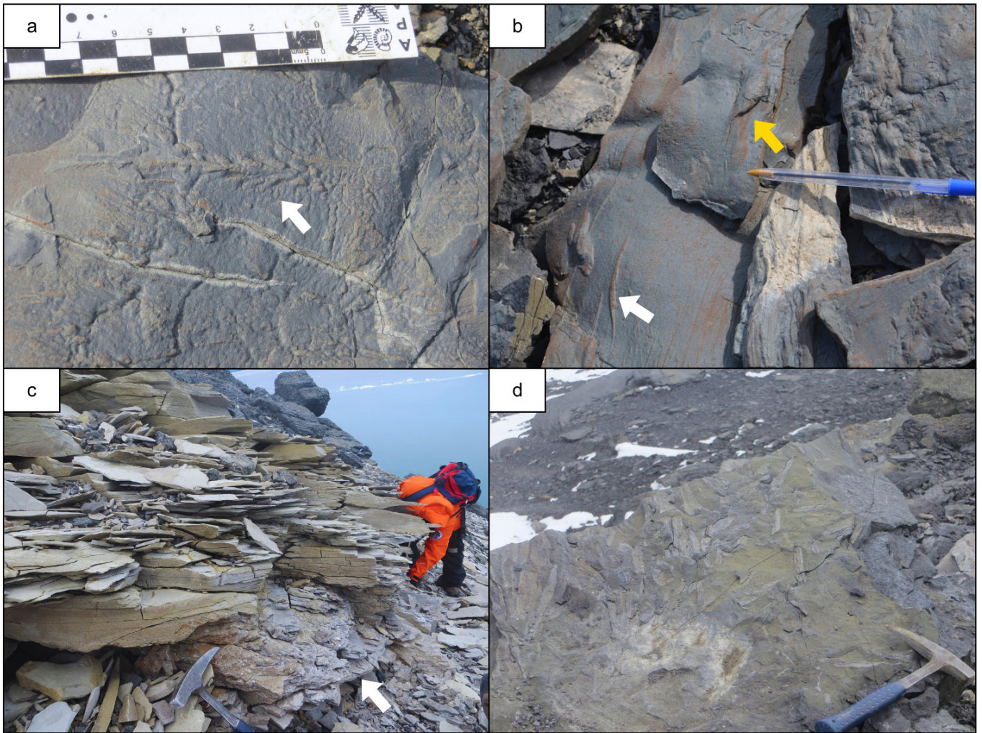
Figura 9. Capas del Miembro La Pera (a) Marcas en chevron en la base del estrato; (b) calco de surco y turboglifo indicados con flecha blanca y amarilla respectivamente en la base de un estrato arenoso, en la sucesión lacustre del Miembro La Pera. (c) Afloramiento de toba/ignimbrita en la parte alta del Miembro La Pera, nótese la base erosiva (flecha) y el arreglo granodecreciente del estrato; (d) Tallos alineados en un nivel de la parte inferior del estrato ilustrado en “c”.
