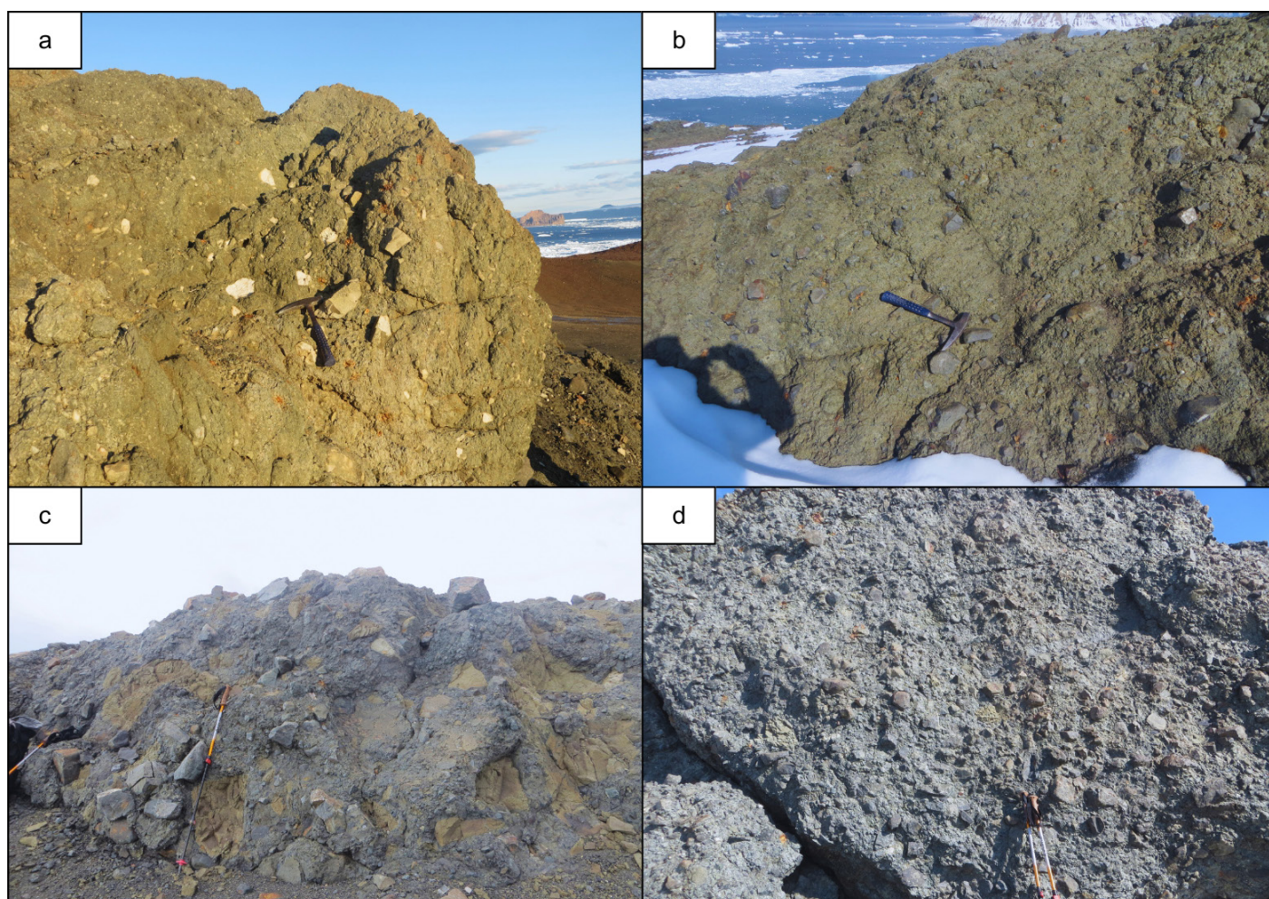
Figura 12. Grupo Volcánico Antarctic Peninsula (a) Brecha piroclástica compuesta de clastos angulosos de rocas volcánicas en una matriz volcánoclastica de lapilli y ceniza; (b) Brecha con clastos redondeados de metarenitas del basamento y clastos angulosos de vulcanitas y tobas en una matriz volcánoclastica; (c) Brecha de bloques de metarenitas del basamento (color gris) y de rocas volcánicas (color castaño); (d) Aglomerado con matriz volcánica y clastos de composición mixta de basamento y vulcanitas.
