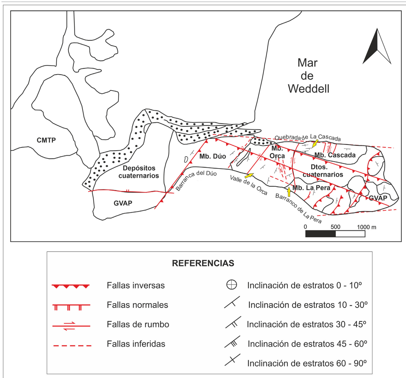
Figura 15. Mapa de detalle de las fallas en la península Camp Hill. GVAP: Grupo Volcánico Antarctic Peninsula.
