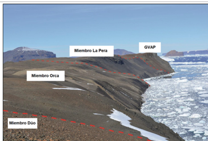
Figura 3. Vista general hacia el este de la costa sur de la península Camp Hill, en la que se observan afloramientos de la parte superior del Miembro Orca y La Pera de la Formación Camp Hill, y hacia el fondo capas del Grupo Volcánico Antártico Península (GVAP).
