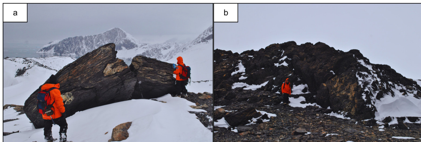
Figura 4. (a) Bloque de procedencia local del basamento del Grupo Trinity Peninsula formando parte de los depósitos morénicos, en el cual se observa el apretado plegamiento típico de la unidad; (b) Afloramiento principal del basamento del Grupo Trinity Peninsula en la península Camp Hill.
