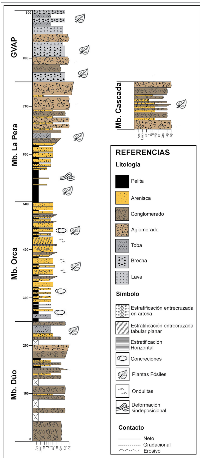
Figura 5. Perfil general de la Formación Camp Hill, y detalle de las subunidades. El Miembro. Dúo presenta barras en sistemas fluviales entrelazados de abanicos aluviales, el Miembro. Orca representaría principalmente un sistema fluvial anastomosado con buen desarrollo de planicie de inundación, cuerpos lacustres menores y barras de desembocadura, y el Miembro. La Pera representa un sistema granocreciente y progradante desde lacustre y luego deltaico hasta abanicos aluviales en sistemas fluviales entrelazados. Las tobas presentes indican actividad volcánica explosiva y esporádica que se vuelve paulatinamente más proximal.
