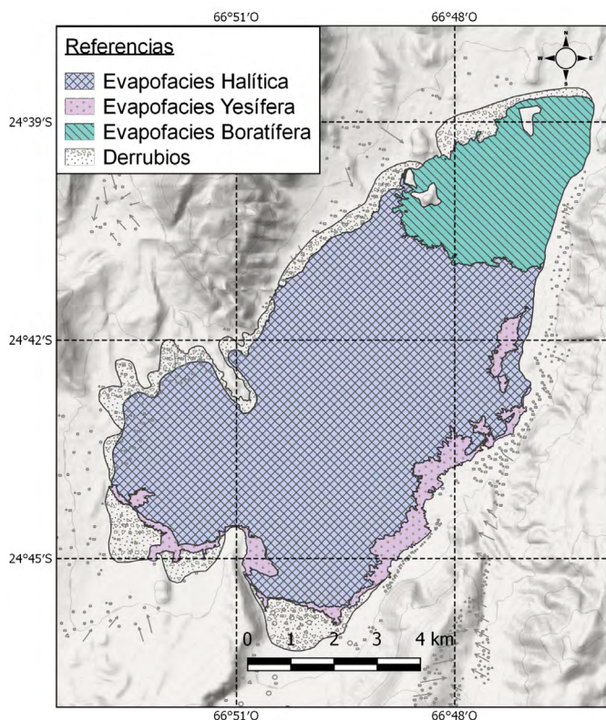
Figura 6. Mapa de zonación de evapofacías dominantes del salar de Pozuelos. Evapofacías boratífera, yesífera y halítica.
