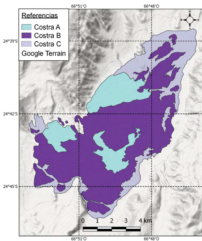
Figura 3. Mapa de costras evaporíticas del salar de Pozuelos (Igarzábal 1996). Costra A: Costra de sal dura poligonada. Costra B: Costra de sal dura rugosa (fósil). Costra C: Costra lisa limosa abrillantada y florecida.
