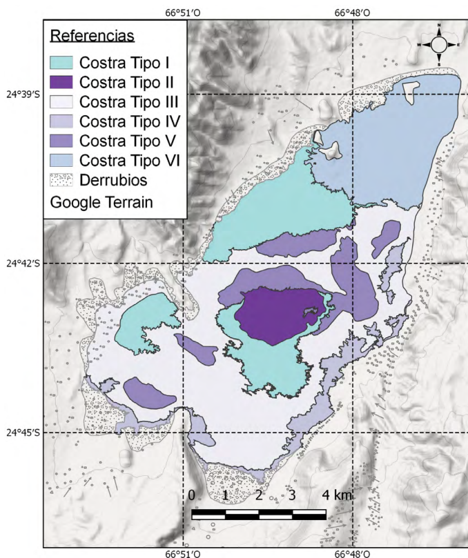
Figura 4. Mapa de costras evaporíticas del salar de Pozuelos (Salta). Tipo I: Costra salina dura lisa. Tipo II: Costra salina dura de alta rugosidad o fósil. Tipo III: Costra salina dura de baja rugosidad. Tipo IV: Costra salina terrosa. Tipo V: Costra salina abrillantada. Tipo VI: Costra salina terrosa asociada a boratos
