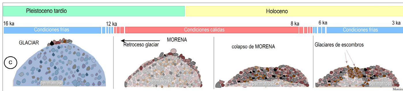
Figura 6. Colapsos de morenas en el valle del río Vacas donde se han desarrollado lenguas de geliflujación y glaciares de escombros criogénicos: a) Imagen Google del sector; a') Fotografía tomada desde helicóptero (S.M. Moreiras); b) Imagen Google del sector; b') Fotografía de la zona tomada desde helicóptero (S.M. Moreiras), y; c) modelo conceptual de los procesos acoplados.
