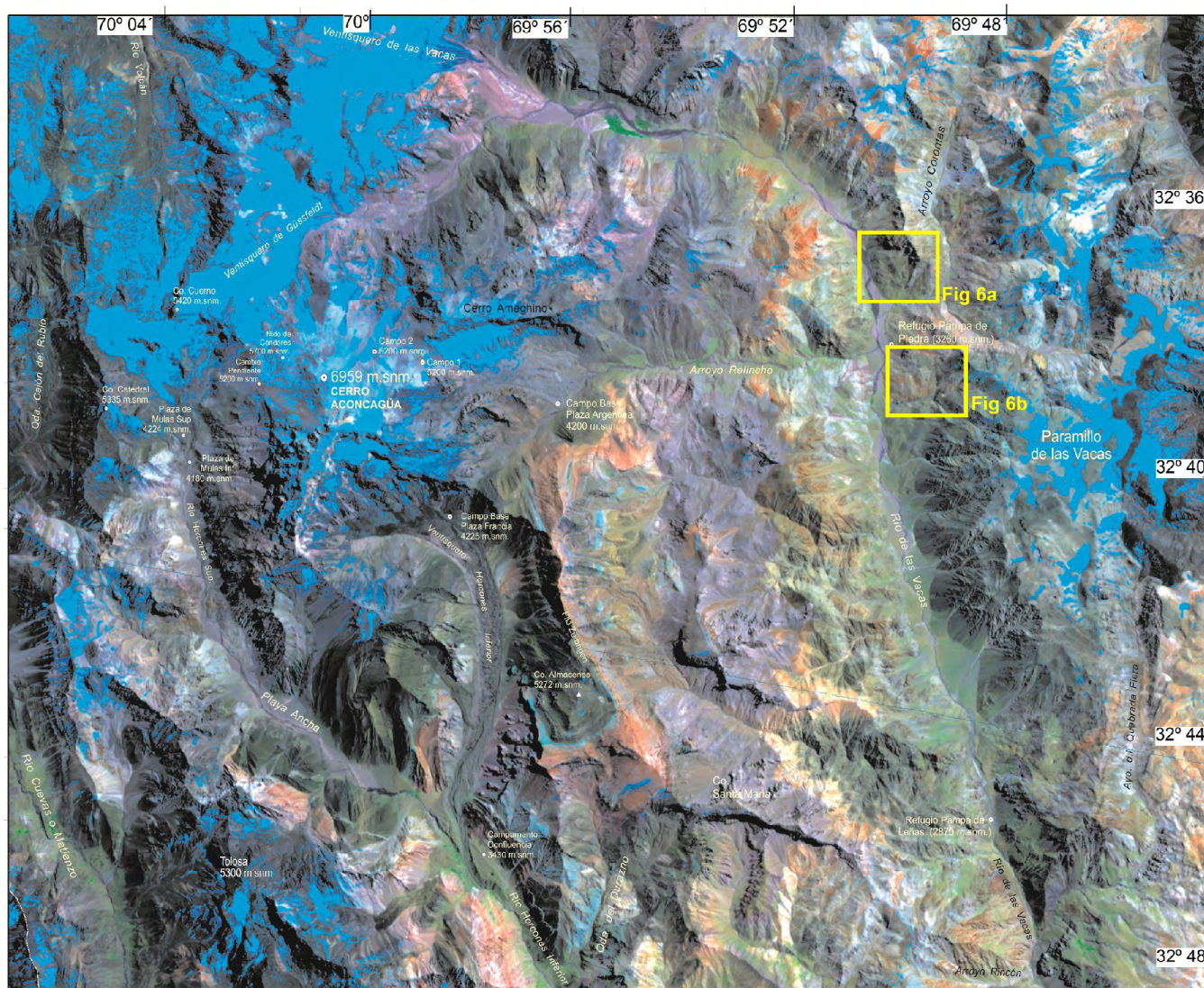
Figura 1. a) Ubicación del parque provincial Aconcagua en el valle del río Mendoza; b) Imagen satelital ASTER (24.03.2003) falso color (RGB 631) de la zona de estudio.
