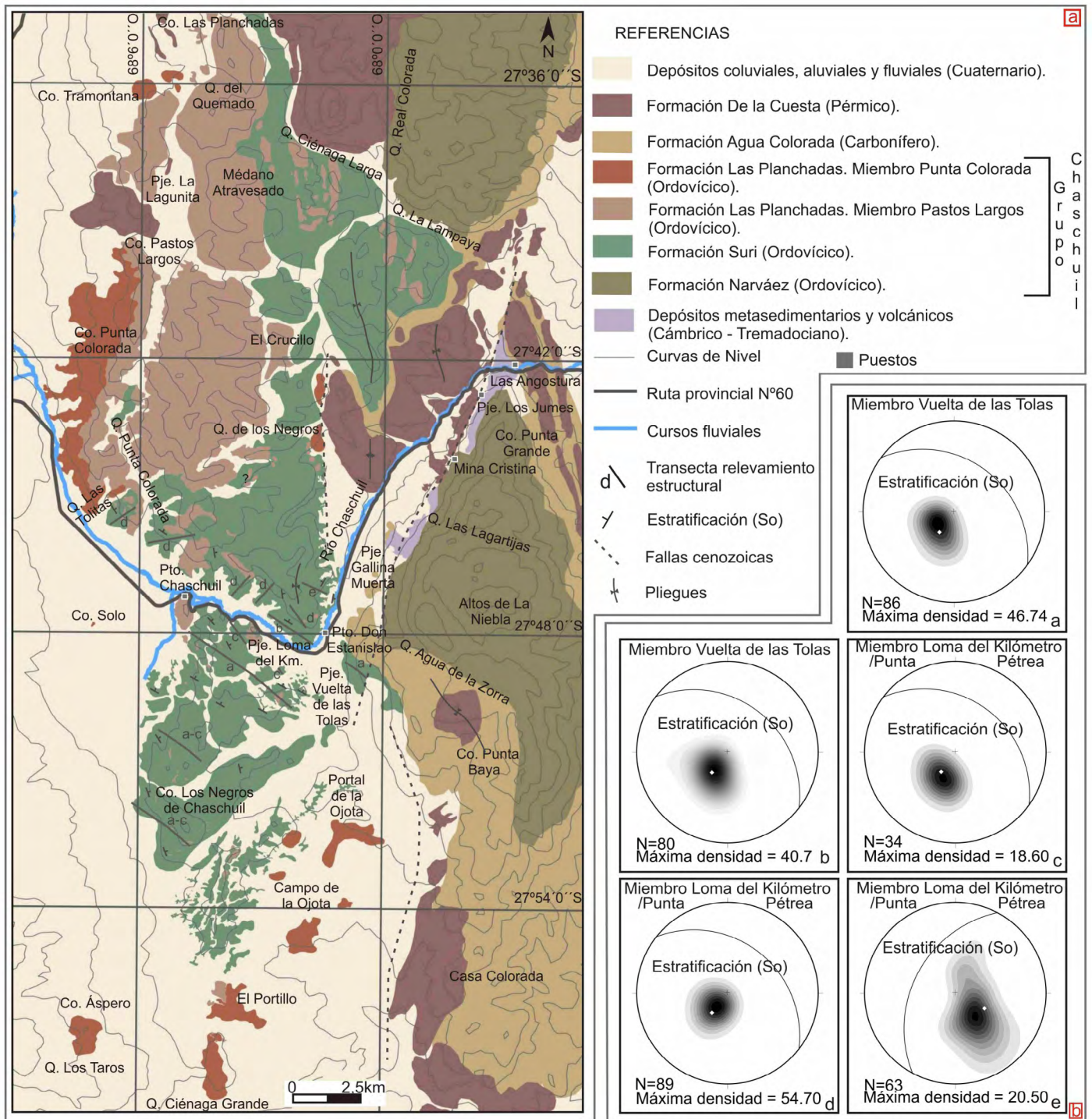
Figura 2. a) Mapa litoestratigráfico del Grupo Chaschuil, donde se representan las diferentes formaciones y miembros que componen la geología del segmento estudiado; b) Representaciones estereográficas del hemisferio inferior de la red de Schmidt, donde se proyectan en diagramas de densidad las orientaciones de la estratificación sedimentaria S_0 relevadas en la Formación Suri. Se proyecta también el polo y plano medio de dicha fábrica.
