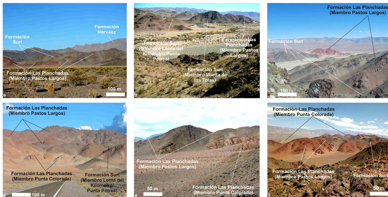
Figura 6. Grupo Chaschuil: a) Foto vista al sureste de las relaciones estratigráficas entre las formaciones del Grupo Chaschuil; b) Foto de los miembros de la Formación Suri en su localidad tipo (vista al suroeste) y su relación con la Formación Las Planchadas; c) Foto del puesto Chaschuil (vista al suroeste), mostrando la intrusividad en la Formación Suri de los domos/criptodomas del Miembro Pastos Largos; d-f) Vista al sur y oeste de la Formación Las Planchadas con la relación estratigráfica de sus miembros; e) La Formación Las Planchadas en la localidad El Portillo; se señala la relación de los miembros plutónicos y volcánicos.
