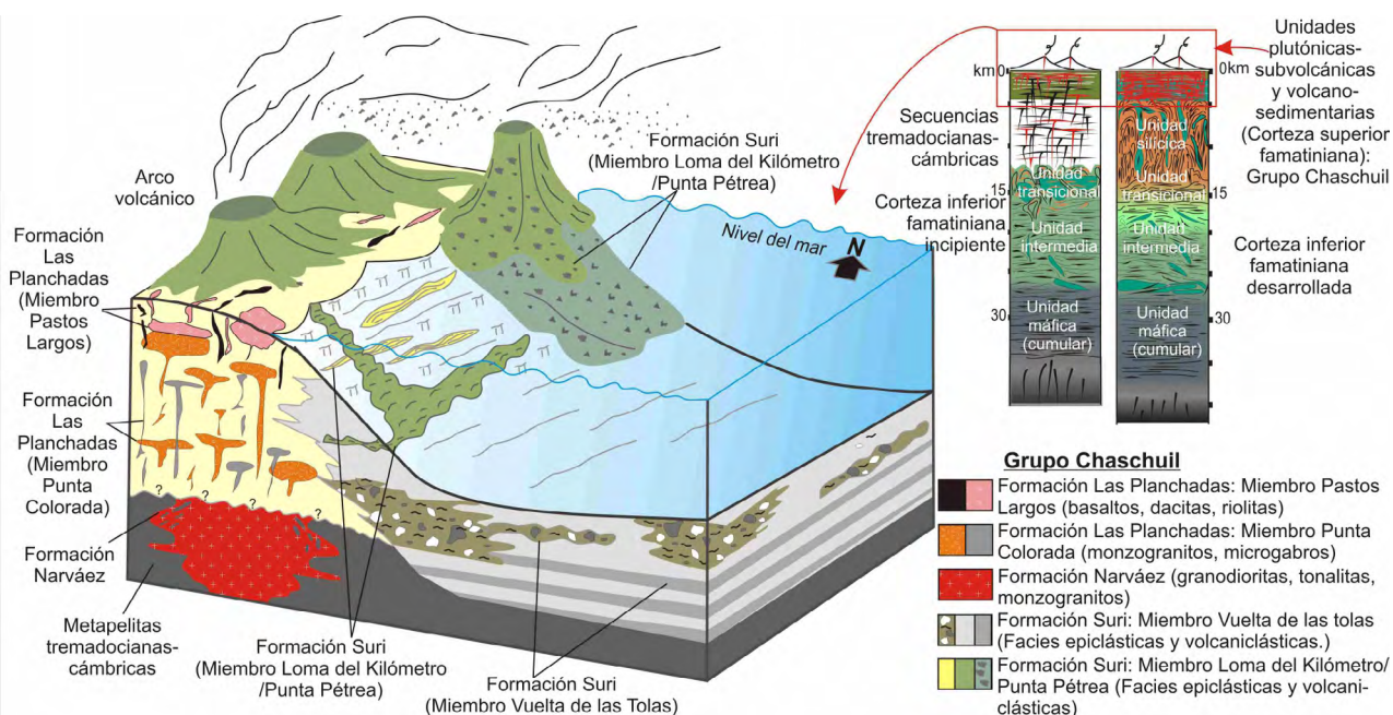
Figura 11. Modelo tridimensional paleogeográfico esquematizado para el arco magmático Famatiniano entre los 27° 27' y 27° 57' latitud Sur (coordenadas actuales), fundamentado en las observaciones realizadas en este trabajo. Modelo basado en Mángano y Buatois (1996), Armas et al. (2017) y Niemeyer et al. (2018). La configuración de la corteza del arco Famatiniano está modificada de Camilletti et al. (2020).
