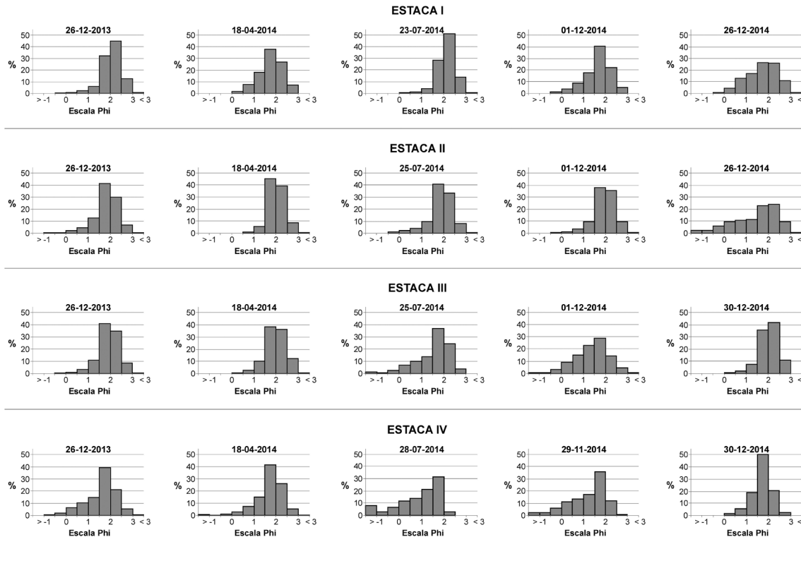
Figura 5: Análisis granulométrico de las muestras colectadas por estaca en playa frontal a lo largo de un año (diciembre 2013 a diciembre 2014). Puede observarse como en la estaca IV predominan las granulometrías más gruesas respecto a las demás sitios.
