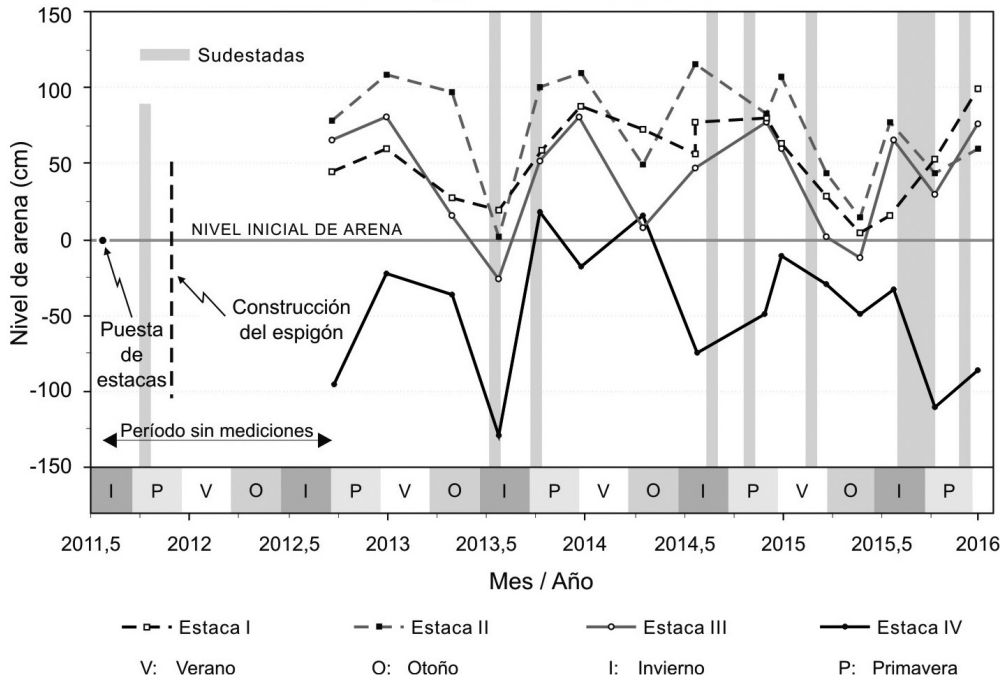
Nivel de arena en playa (Camet Norte - Mar de Cobo) Período julio 2011 - diciembre 2015
