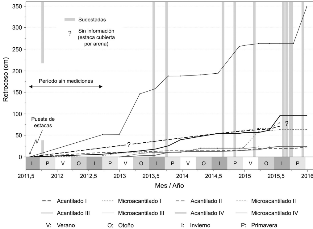
Retroceso del acantilado y microacantilado (Camet Norte - Mar de Cobo) Período julio 2011 - diciembre 2015
