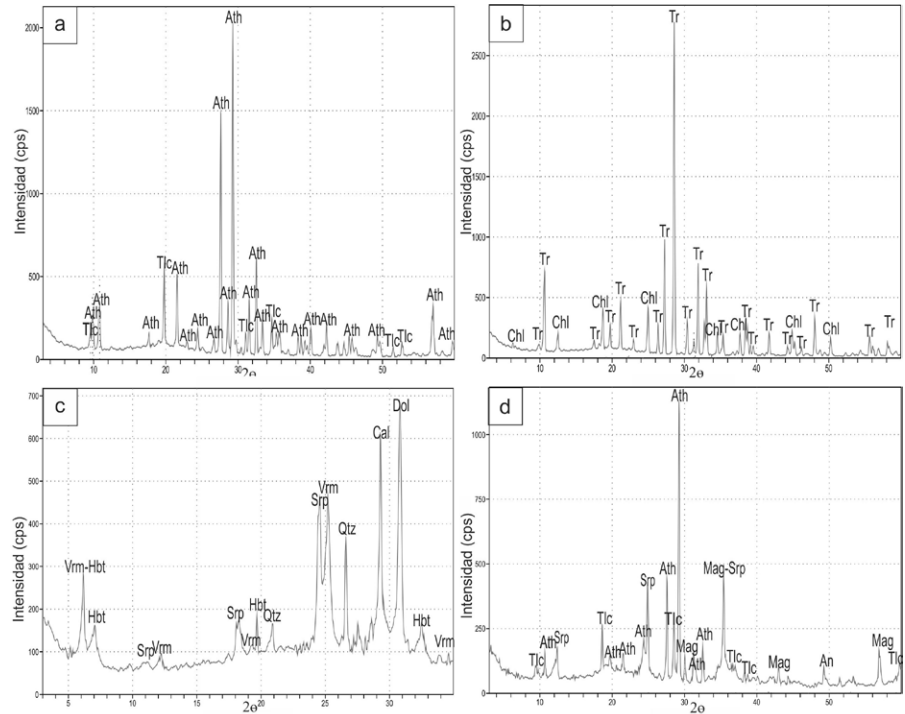
Figura 5: a) Difractograma de las vetillas (Ath: antofilita, Tlc: talco) de la mina La Isla; b) Difractograma de la roca de caja anfibolítica (Tr: tremolita, Chl: clorita) de la mina La Isla; c) Difractograma de la zona de vermiculita de la mina Mauro (Vrm: vermiculita, Hbt: hidrobiotita, Srp: serpentina, Qtz: cuarzo, Cal: calcita, Dol: dolomita); d) Difractograma de minerales en vetillas en la roca de caja de la mina Mauro (Tlc: talco, Ath: antofilita, Srp: serpentina, Mag: magnetita).
