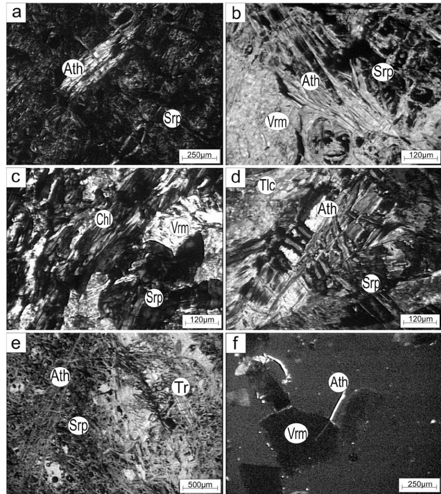
Figura 3: Mina Mauro. a) Fotomicrografía con analizador intercalado de un cristal de antofilita (Ath), en una masa de serpentinita (Srp); b) Fotomicrografía sin analizador intercalado de cristales aciculares astillosos de antofilita (Ath) en contacto con un relicto de serpentinita (Srp) y una masa de vermiculita (Vrm); c) Fotomicrografía con analizador intercalado de islotes de vermiculita (Vrm) y clorita magnesiana (clinocloro) (Chl) en la serpentinita (Srp); d) Fotomicrografía con analizador intercalado de grandes cristales de tremolita (Tr) en una masa de talco (Tlc), conservándose relictos de la serpentinita (Srp); e) Fotomicrografía sin analizador intercalado de minerales opacos diseminados en la serpentinita (Srp) con largos y finos cristales de antofilita (Ath) y tremolita (Tr); f) Fotomicrografía con analizador intercalado de fibras largas y flexuradas de antofilita (Ath) en la vermiculita (Vrm).
