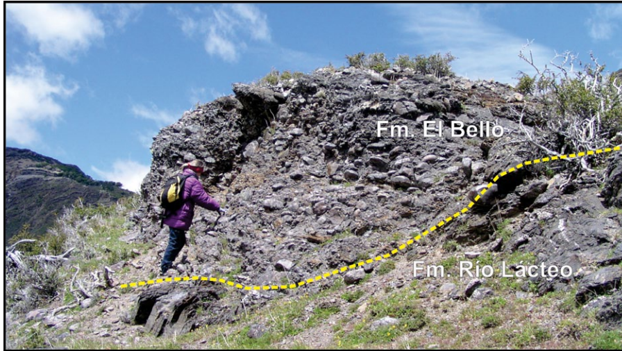
Figura 3: Superficie basal de la Formación El Bello, labrada en la Formación Río Lácteo. Al fondo a la izquierda se observa el cerro Pirámide, donde continúa el perfil tipo de esta unidad.
