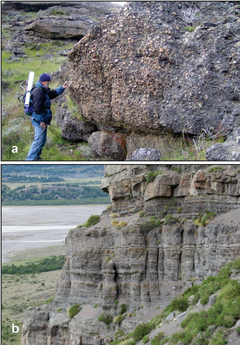
Figura 4: a) Detalle del aspecto de los conglomerados en la sección tipo de la Formación El Bello, cerro Pirámide. b) Vista hacia el este de la sección media del perfil tipo de la Formación El Bello en el cerro Pirámide. Nótese la alternancia cíclica de conglomerados, areniscas y pelitas. Al fondo, el río Mayer.
