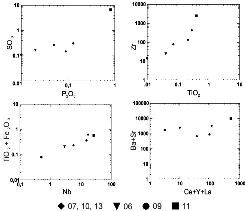
Figura 6: Relaciones (TiO_2 + Fe_2O_3) vs. (Cr+Nb) , Zr vs. TiO_2 , y (Ba + Sr) vs. (Ce+Y+La) .
