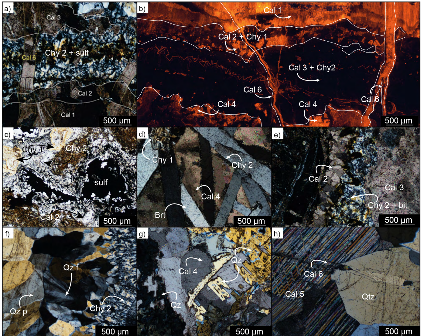
Figura 11. Minerales de ganga presentes en vetillas y brechas de Valle Esperanza: a) Venilla crustiforme con calcita 1-3, brechada y cementada por calcedonia 2 con inclusiones de sulfuros, cortadas por calcita 6; b) Imagen de catodoluminiscencia que muestra relación textural de calcitas 1, 2, 3, 4 y 6; c) Calcita 2 euhedral, calcedonia 1 coliforme y sulfuros brechados e incorporados por calcedonia 2; d) Baritina tabular incorpora agregados de calcedonia 1; calcita 4 rellena intersticios; calcedonia 2 corroe bordes de baritina y calcita 4; e) Calcita 2 y calcita 3 brechadas por calcedonia 2 con inclusiones de bitumen; f) Calcedonia 2 fibrosa en bandas coliformes, bandas de cuarzo flameante y cuarzo plumoso; g) Baritina con reemplazo total de cuarzo; calcita 4 rellena intersticios; h) Calcita 5 rellena oquedades de cuarzo; microvetillas de calcita 6 cortan a cuarzo y calcita 5. Cal: calcita, Chy: calcedonia, Qtz f: cuarzo con textura flameante, Qtz p: cuarzo con textura plumosa, Sulf: sulfuros y sulfosales, bit: bitumen.
