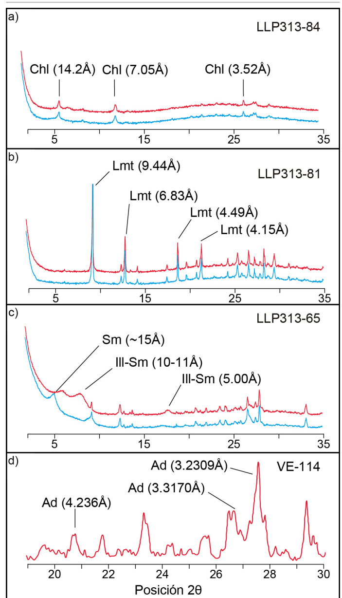
Figura 13. Difractogramas de rayos X con los picos característicos de los minerales secundarios identificados. En rojo se muestran los análisis realizados en muestras secadas al aire y en azul las saturadas en etilenglicol. a) Chl: Clorita; b) Lmt: Laumontita; c) Ill-Sm: Interstratificado illita-esmectita y Sm: esmectita; d) Ad: Adularia.
