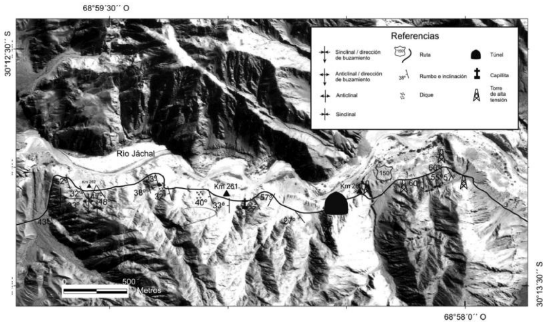
Figura 9: Esquema realizado sobre un mosaico ortorestituido mostrando los datos de rumbo e inclinación y las principales estructuras identificadas en el perfil de la sierra de los Túneles (Tomada de Azcurra, 2007).
